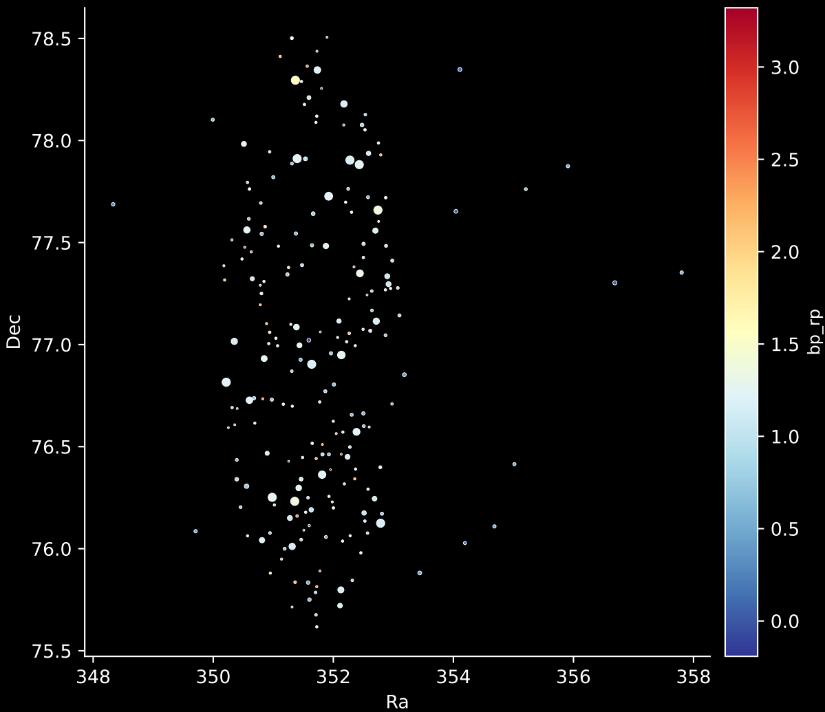
APOGEE DR17 Field: [CVZ_OB01_btx] Stars: 211
