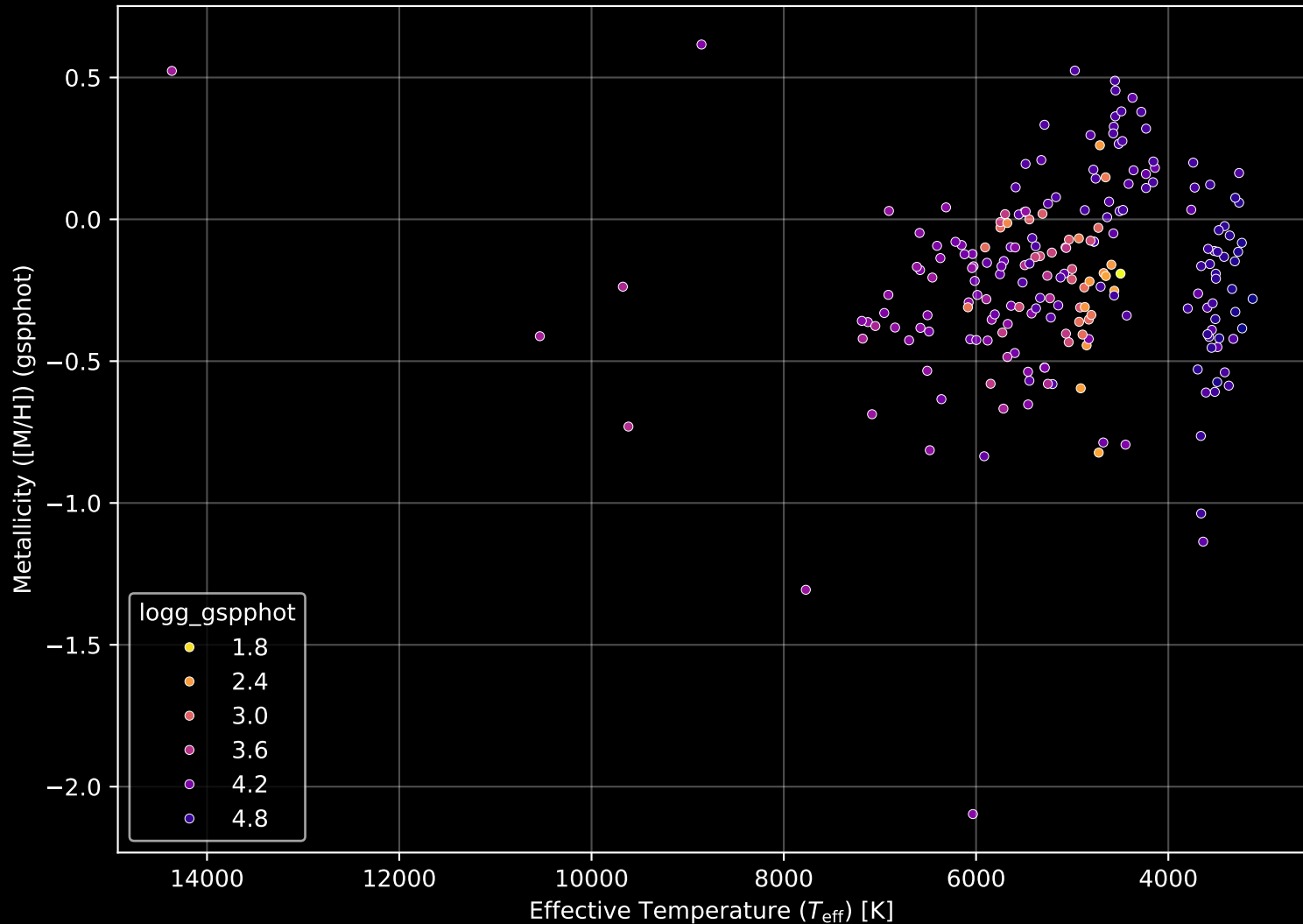
APOGEE DR17 Field: [CVZ_OB01_btx] Stellar Population Parameters (n= 211)
